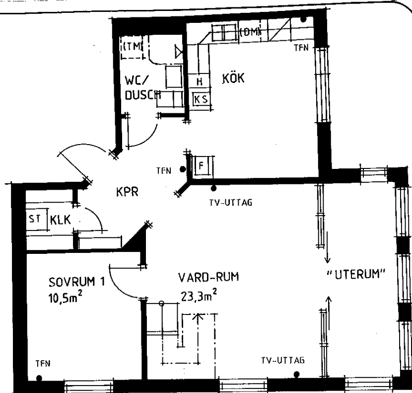
PLAN 3 TRAPPOR
