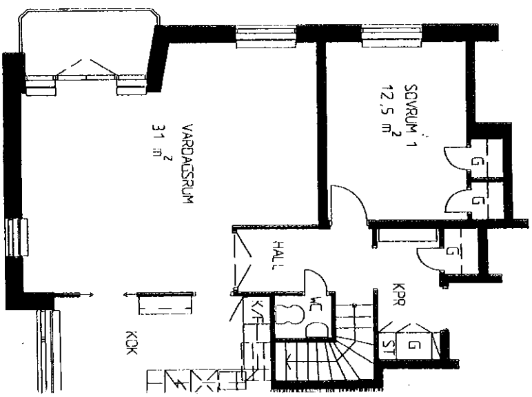
NEDRE PLAN
