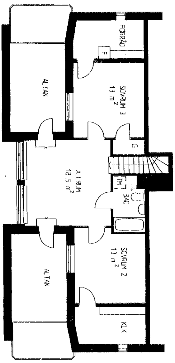
ÖVRE PLAN
